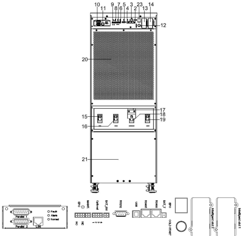
Рисунок 2 — Общий вид задней панели изделия, где
