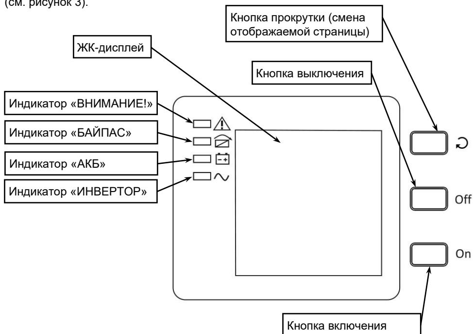
Рисунок 3 — ЖК-дисплей
